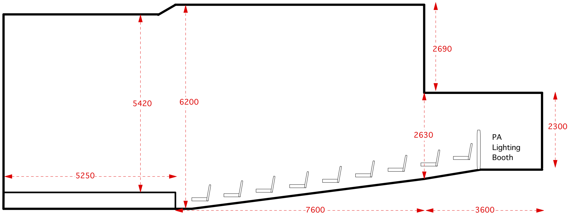
Kitty Hall 会場断面図 Scale 1/70
