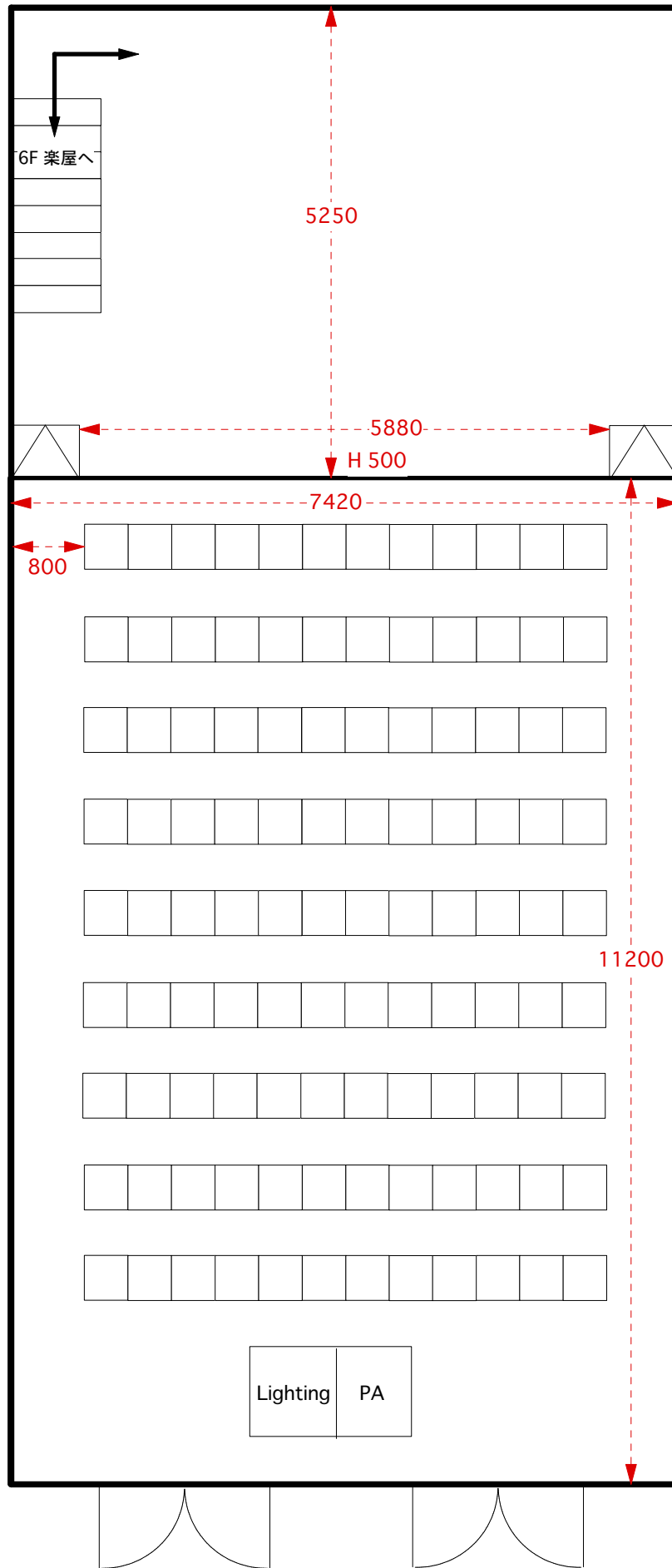
Kitty Hall 会場平面図 Scale 1/70
